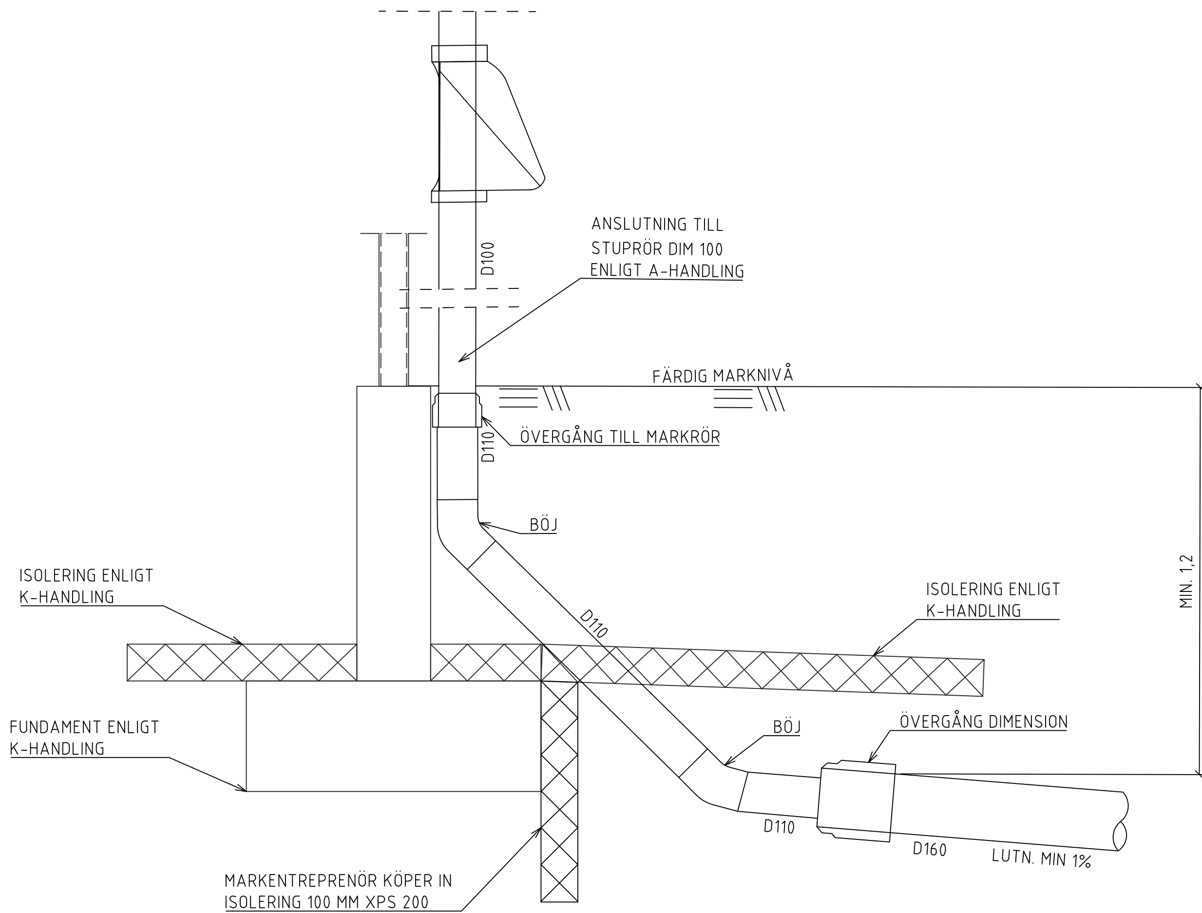
DETALJ ANSLUTNING, SR3, MARKANSLUTNA STUPRÖR MOT DIM 100
