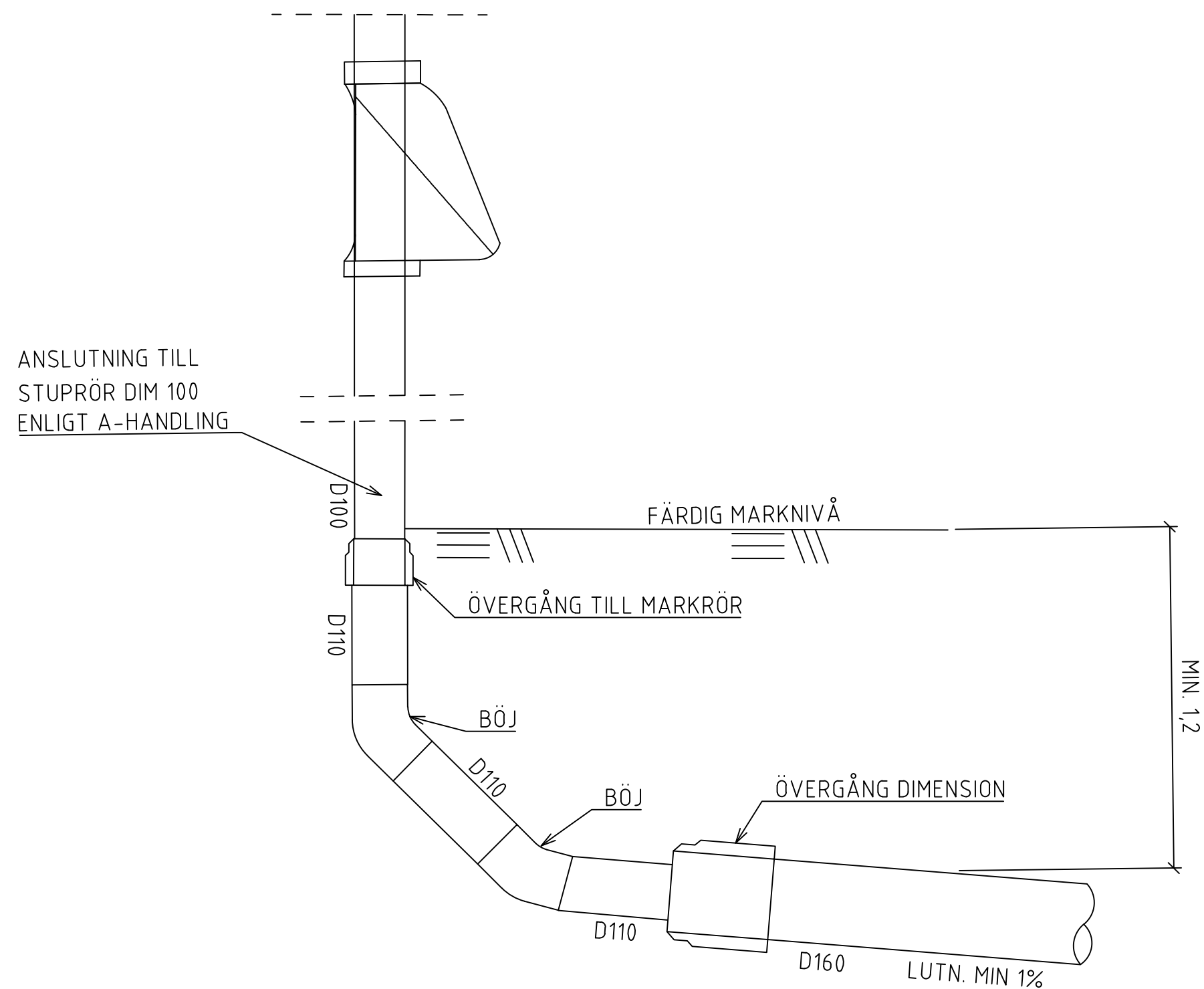
DETALJ ANSLUTNING, SR1, MARKANSLUTNA STUPRÖR MOT DIM 100
