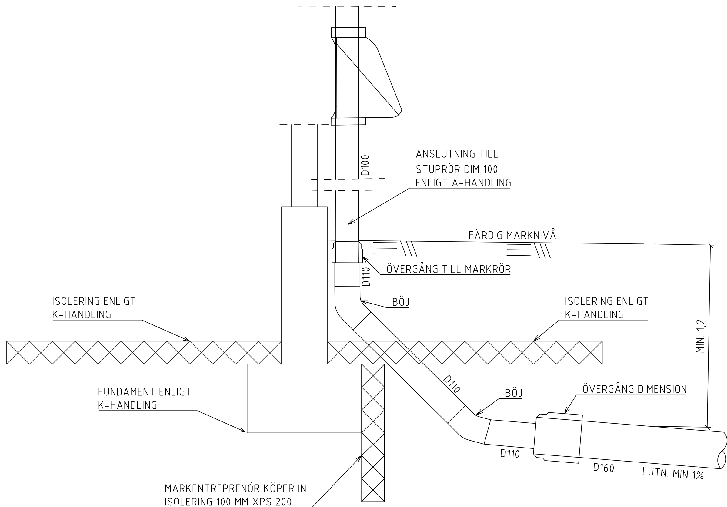
DETALJ ANSLUTNING, SR4, MARKANSLUTNA STUPRÖR MOT DIM 100
